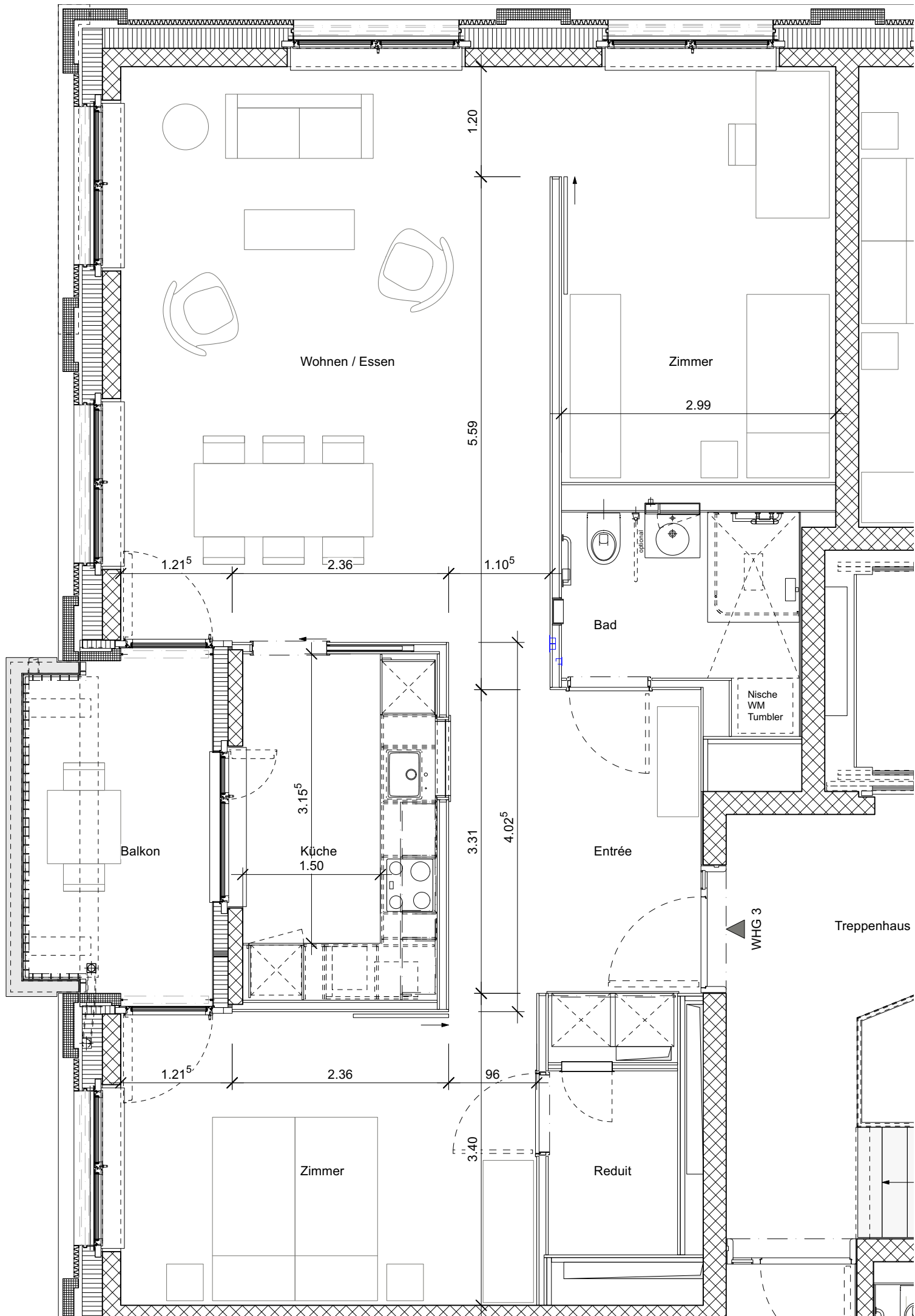
Grundriss Wohnung 3_ 1:50
