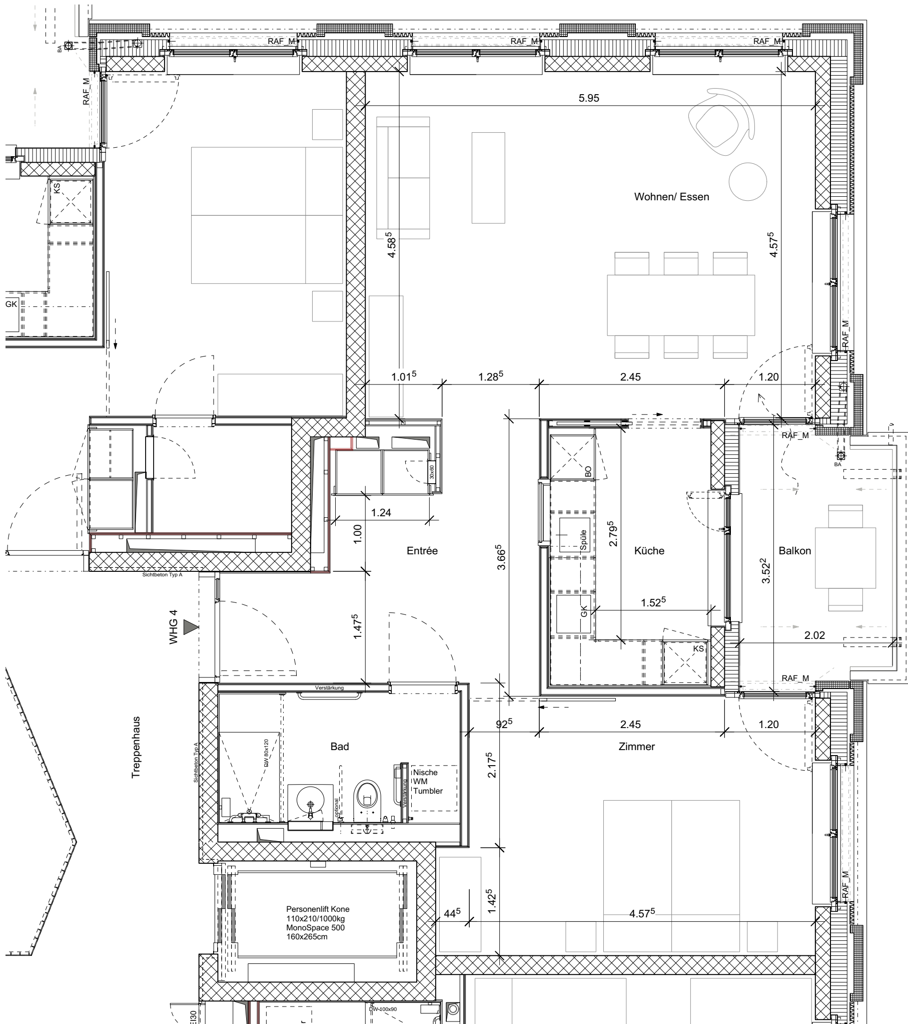
Grundriss Wohnung 4_ 1:50
